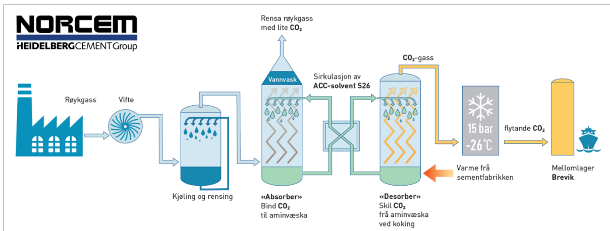
Figur 4.3 Illustrasjon av CO 2 -fangstprosessen ved Norcem
