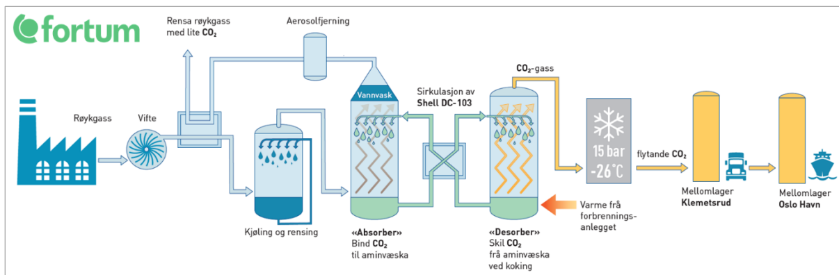
Figur 4.5 Illustrasjon av CO 2 -fangstprosessen ved Fortum Oslo Varme
