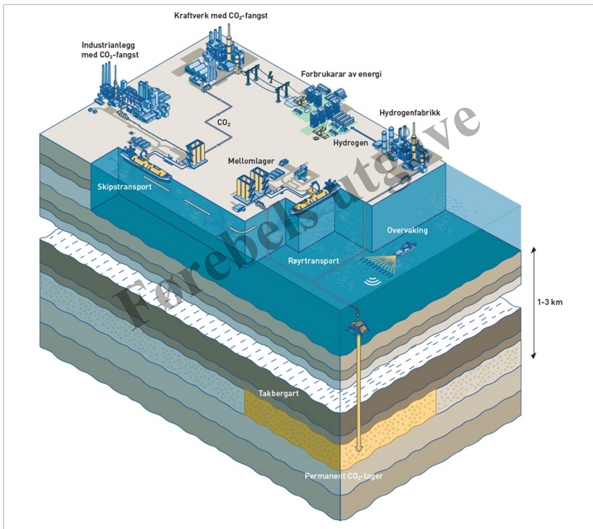
Figur 2.1 Illustrasjon av CO 2 -fangst frå ulike industrianlegg og kraftproduksjon, transport i rør og med skip, geologisk lagring av CO 2
