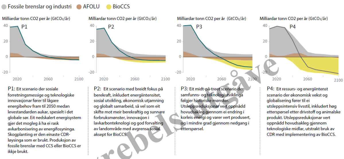
Figur 2.3 Fordeling av bidrag til globale netto utslepp av CO 2 i fire illustrasjonar av modellerte utsleppsbanar
